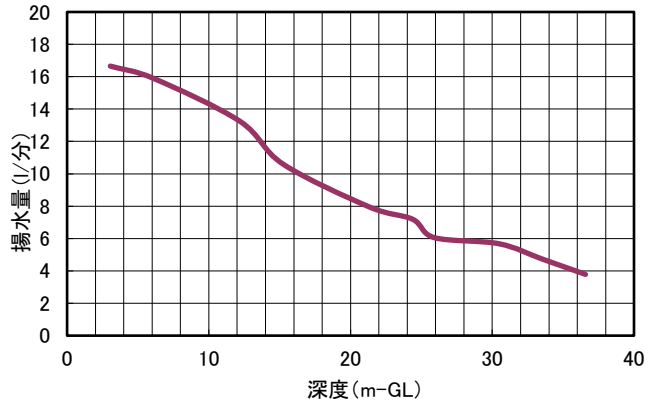
MONSOON 性能曲線
