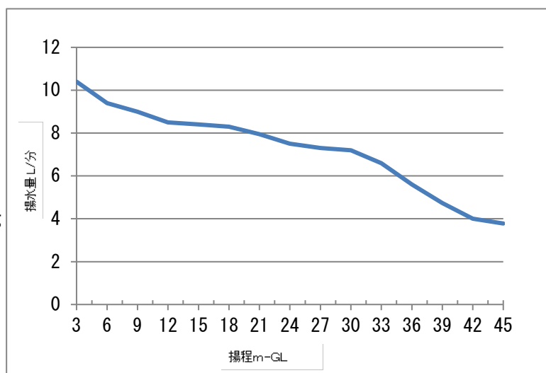
ハリケーンポンプ性能曲線
