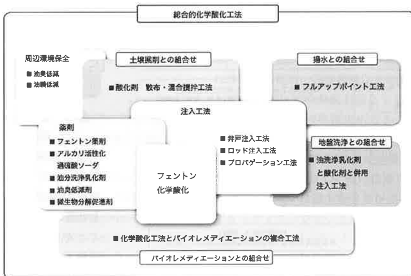
第1図 総合的にフェントン化学酸化工法と構成する要素技術
